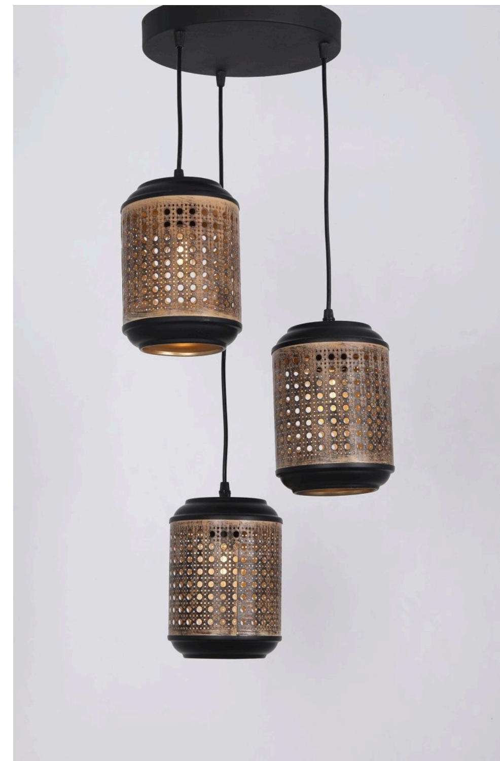
Item No : DRL 10584-3 Lamp : 3XE27 Size : D320MM X H1400MM Finish : Black + Rustic Gold Material : Metal
